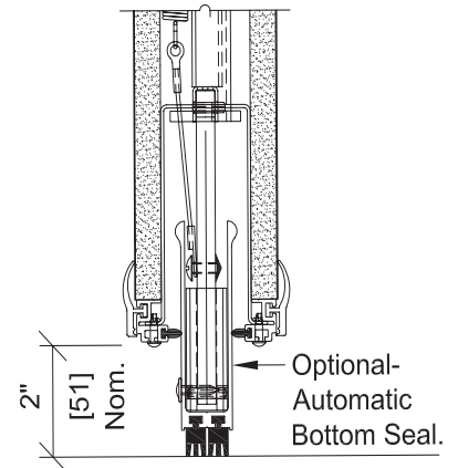
Optional Automatic Bottom Seal
